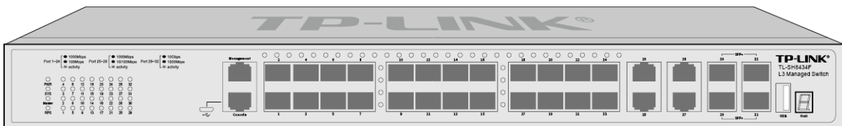
图 2-3 TL-SH8434F 前面板
