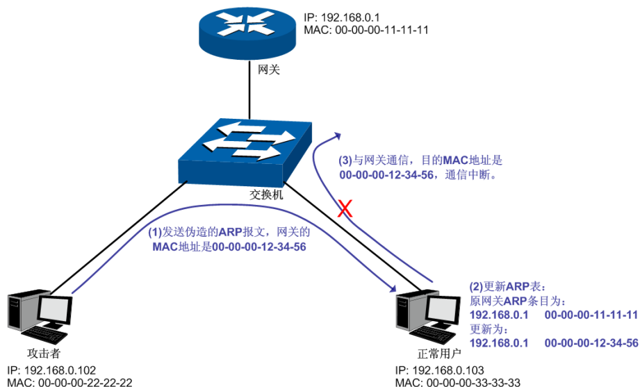
图 13-11 ARP 攻击-网关仿冒示意图
